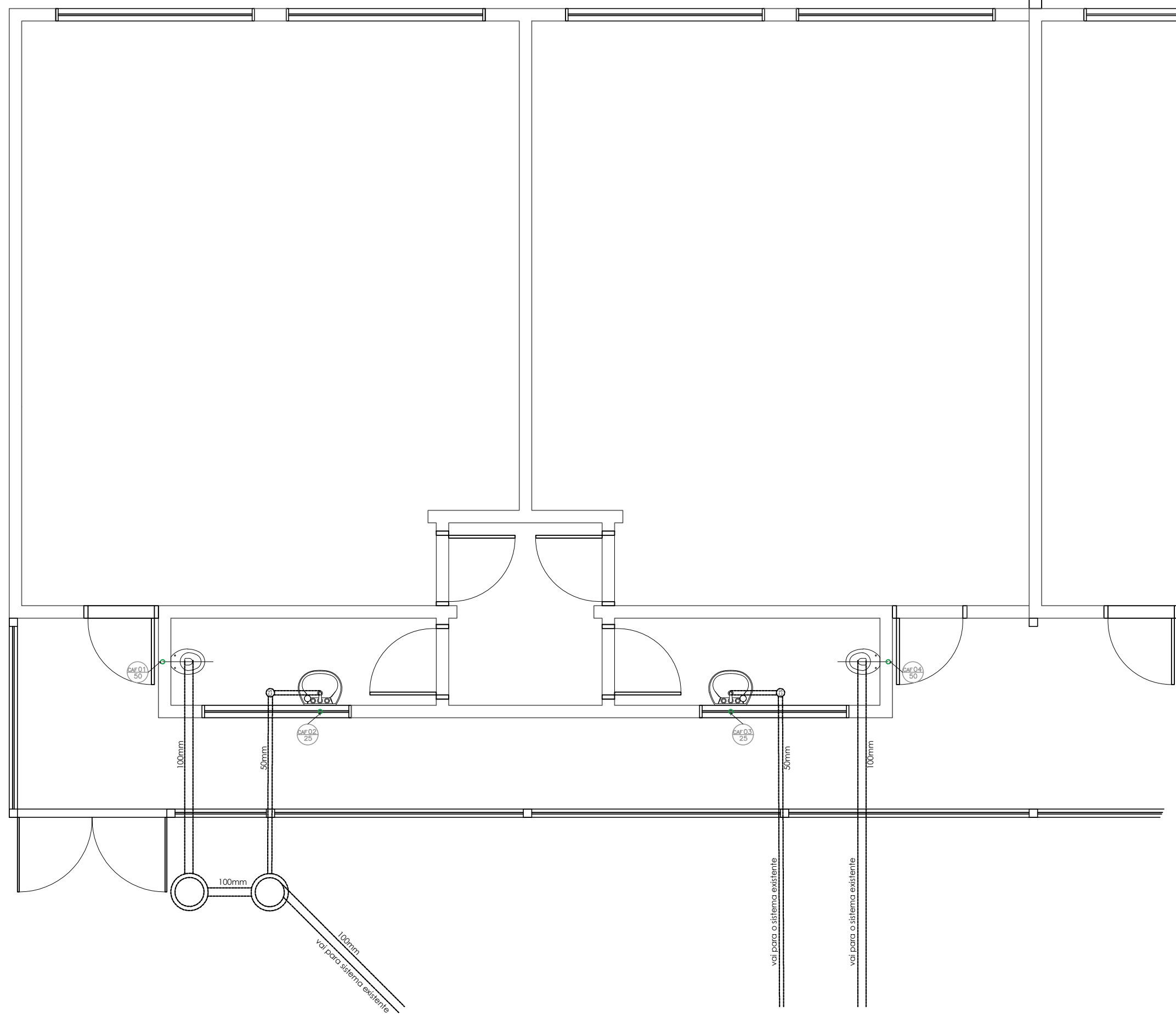
Projeto Hidrossanitário Esc. 1:50
