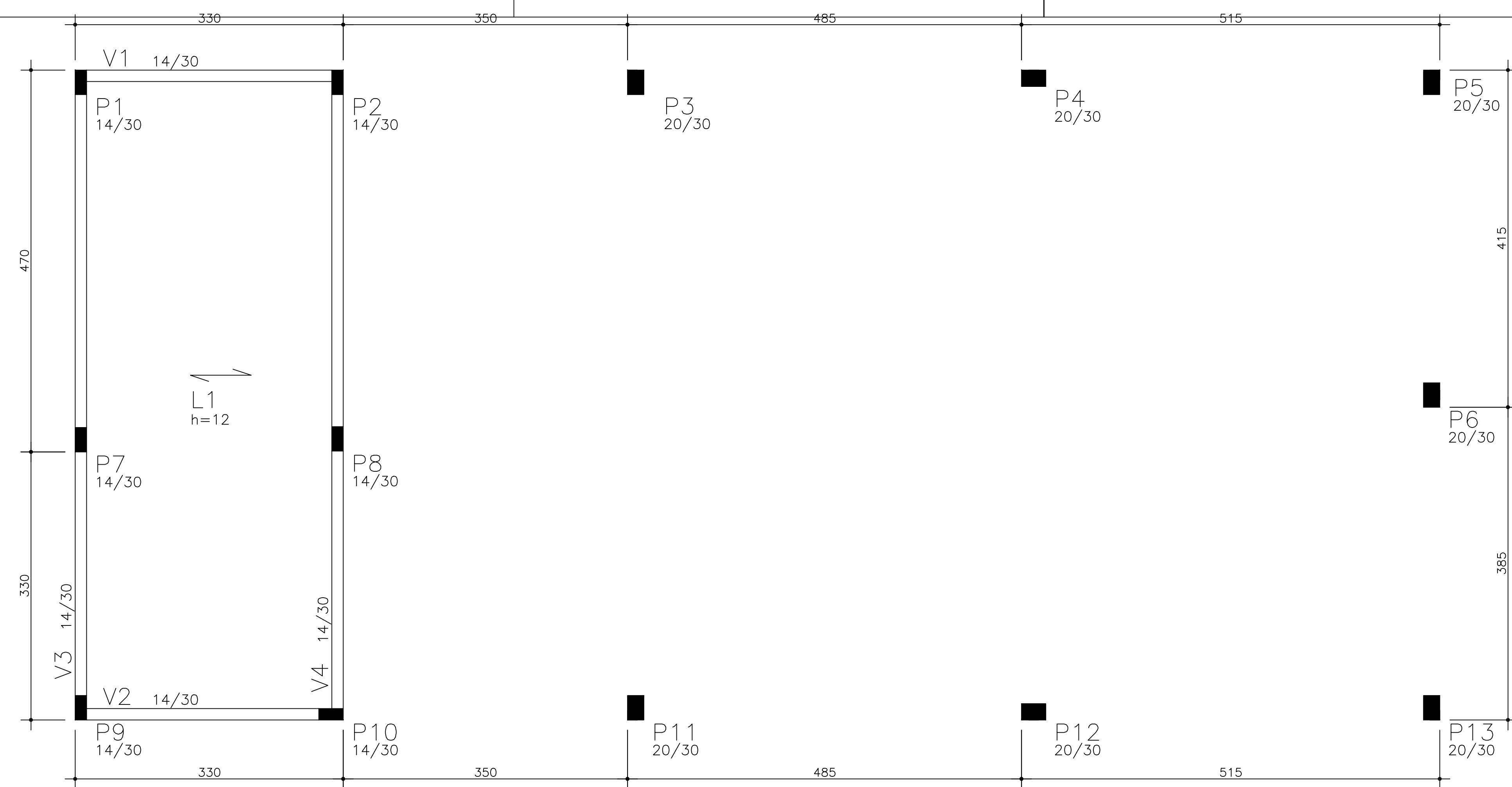
PLANTA DE FORMA PAVTO. COBERTURA 02
