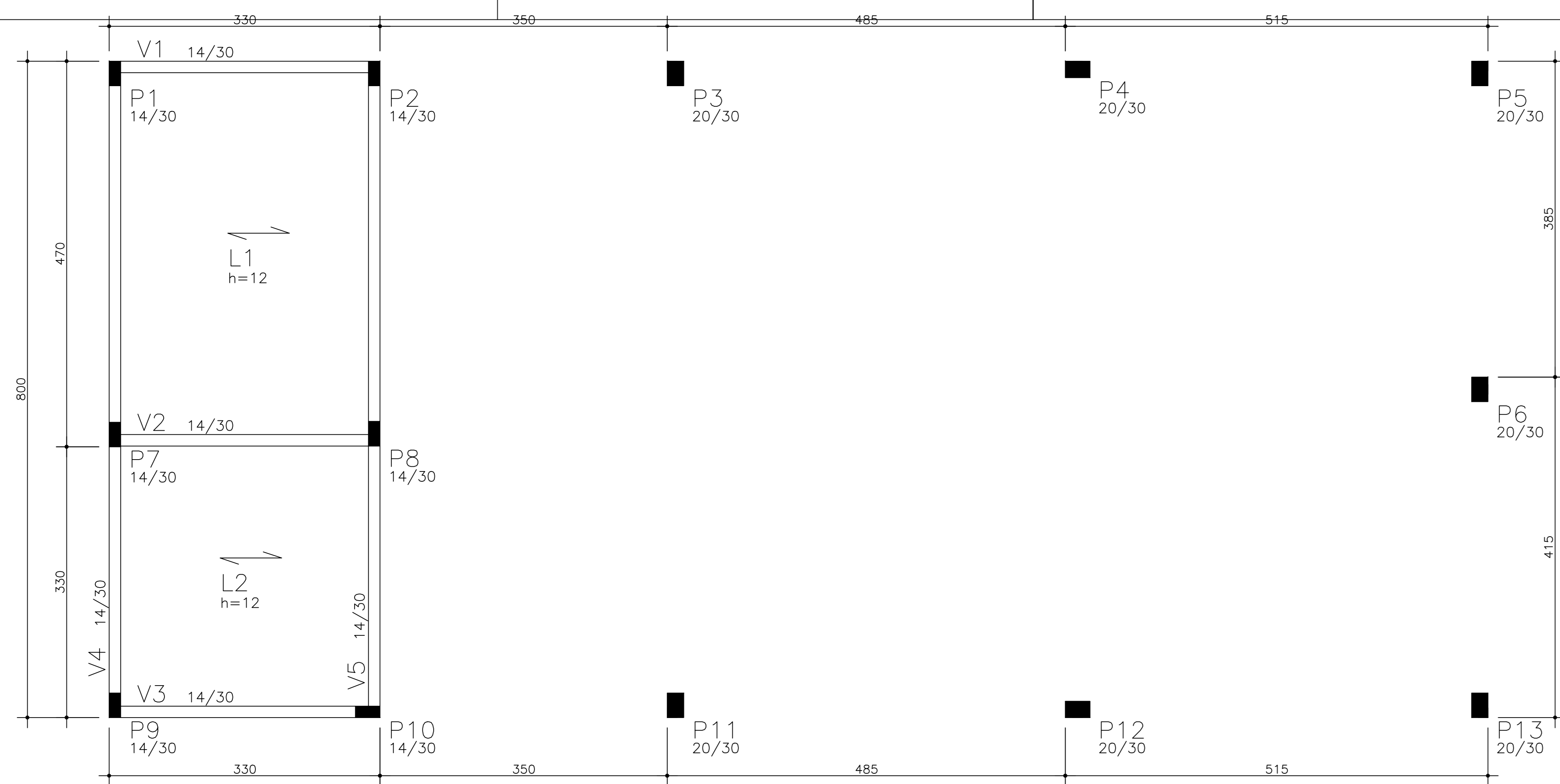
PLANTA DE FORMA PAVTO. MEZANINO
