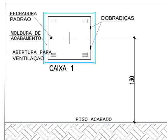
DETALHE QUADRO DE DISTRIBUIÇÃO PARA TELEFONIA E LÓGICA
