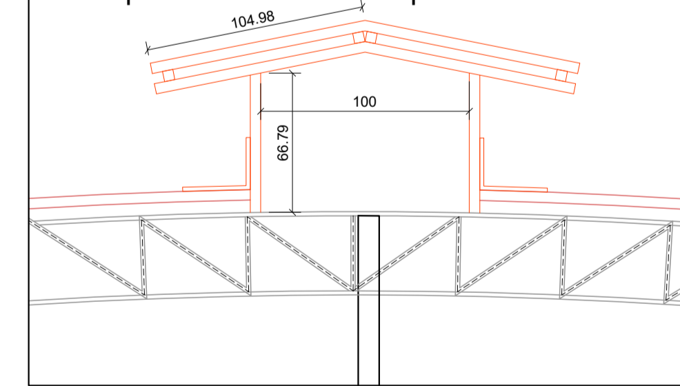
DETALHE VENTILAÇÃO ESC: 1/25
