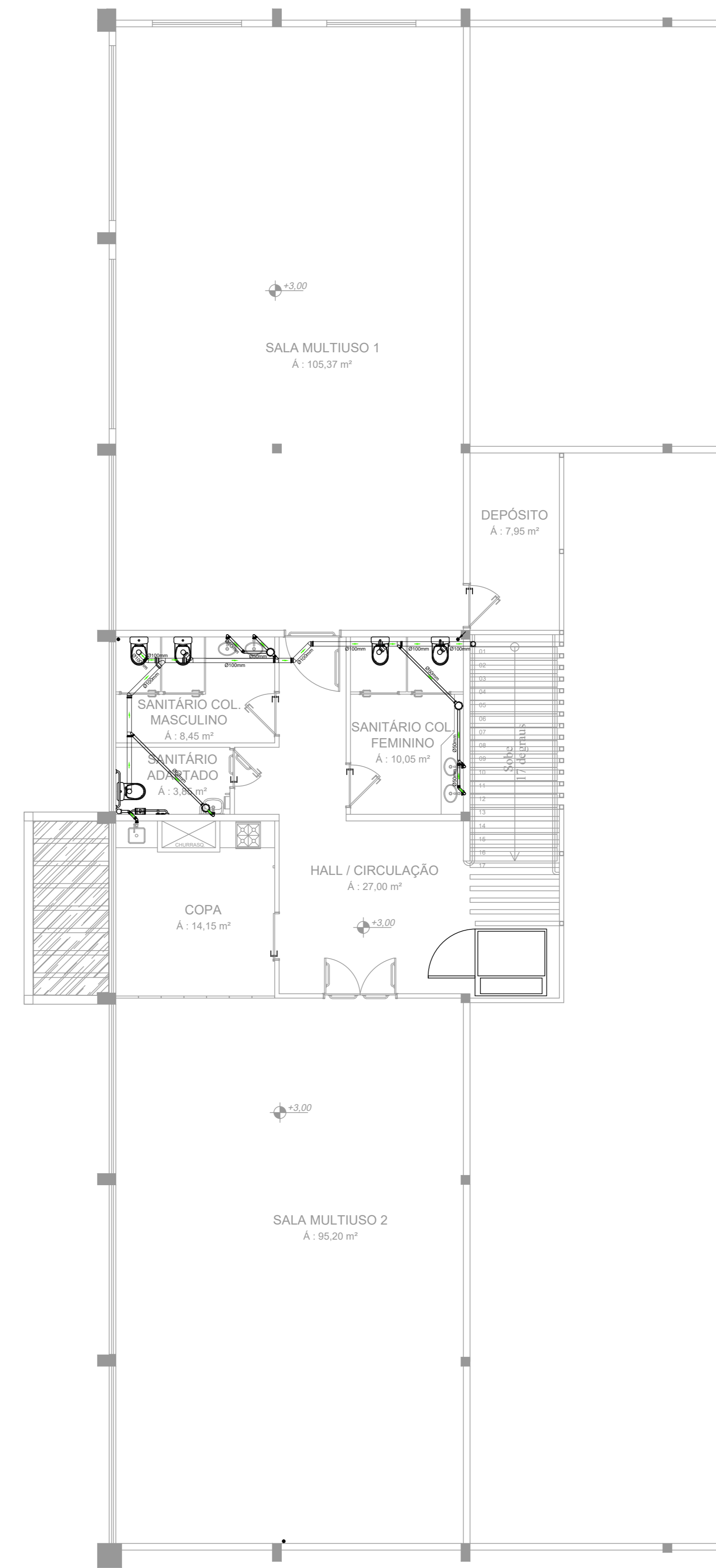
SANITÁRIO SUPERIOR ESC: 1/75
