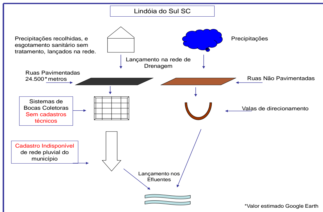
Figura 58 - Fluxograma do sistema de drenagem
