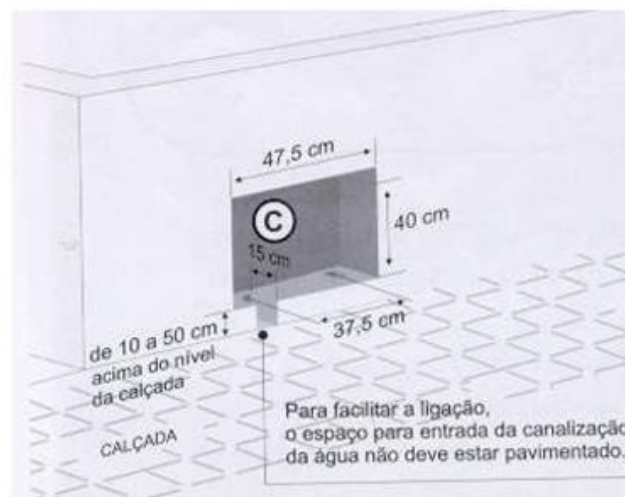
Figura 49 - Dimensões de abrigo para instalação do Micromedidor
