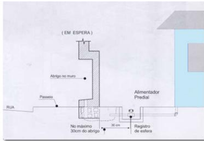
Figura 48 - Corte padrão de entrada de água
