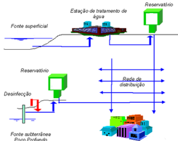
Figura 1 – Sistema de Abastecimento de Água Fonte: Águas do Amazonas (2010)
