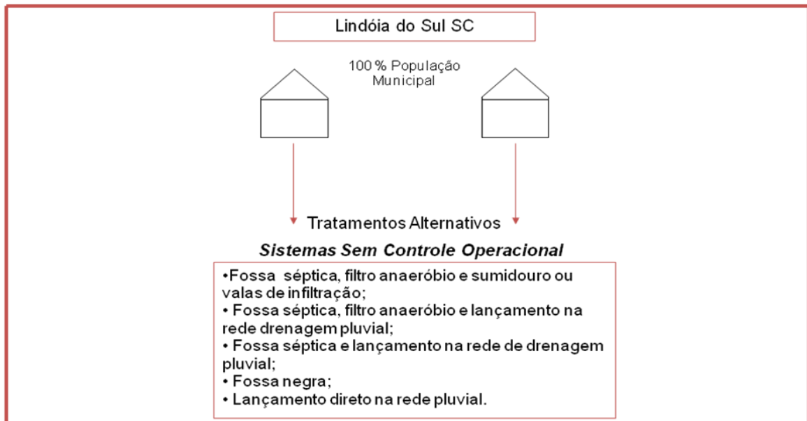
Figura 51 - Fluxograma de Caracterização dos Sistemas Alternativos de Tratamento de Esgoto Sanitário do Município
