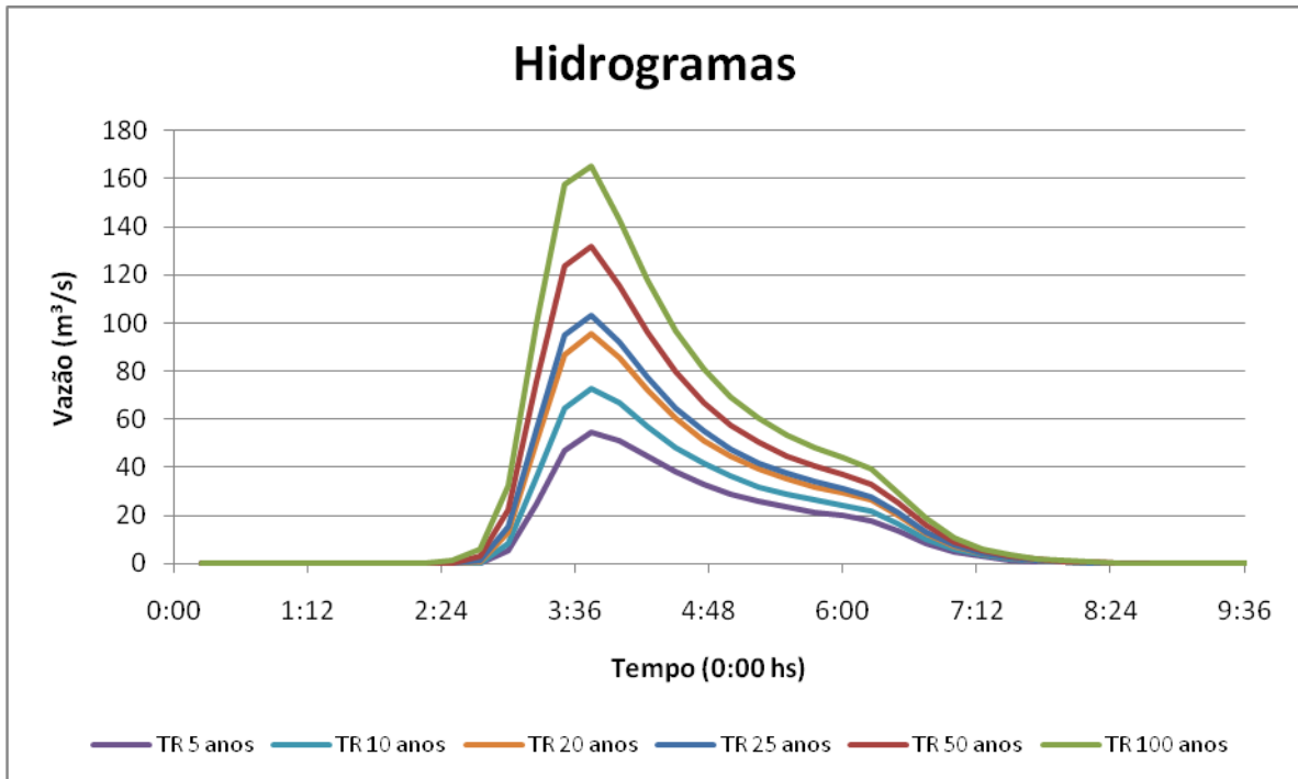
Figura 57 - Hidrogramas de Cheias
